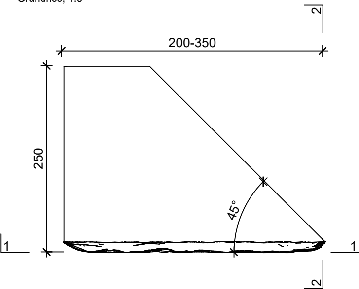
Grundriss, 1:5
