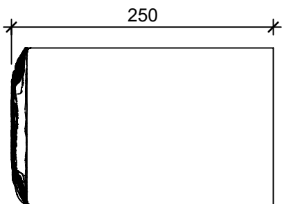
Schnitt 2-2, 1:5
