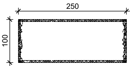
Schnitt 2-2, 1:5
