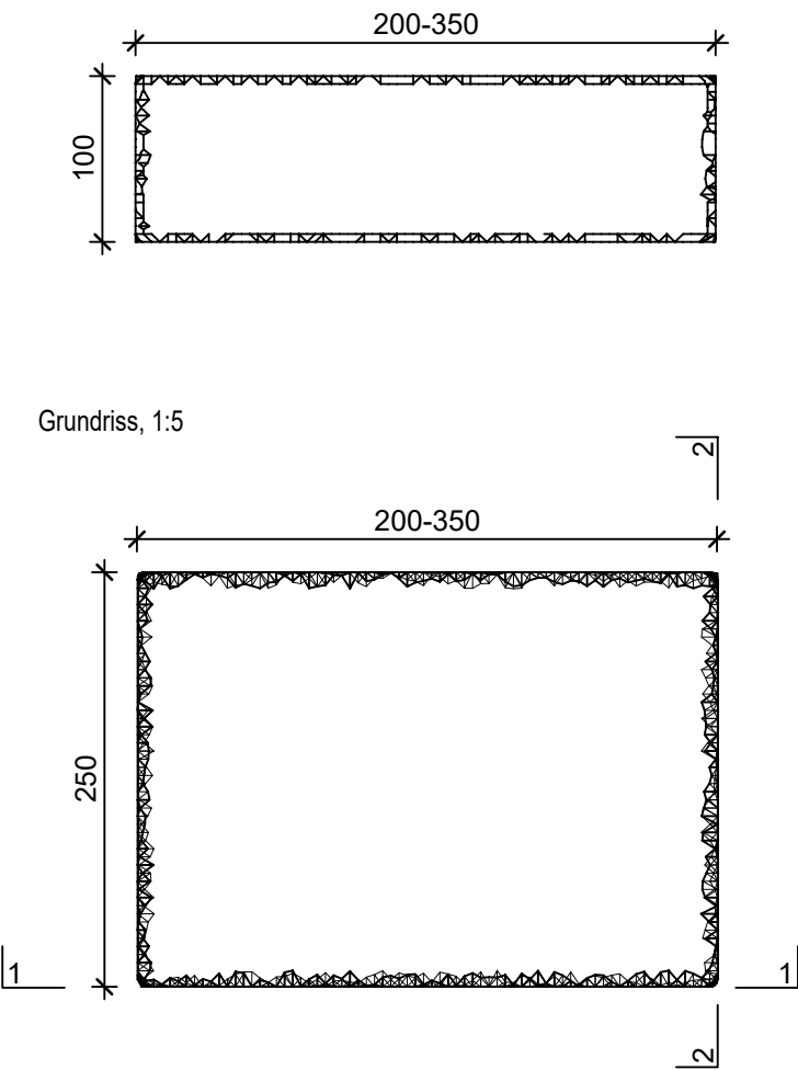
Schnitt 1-1, 1:5
