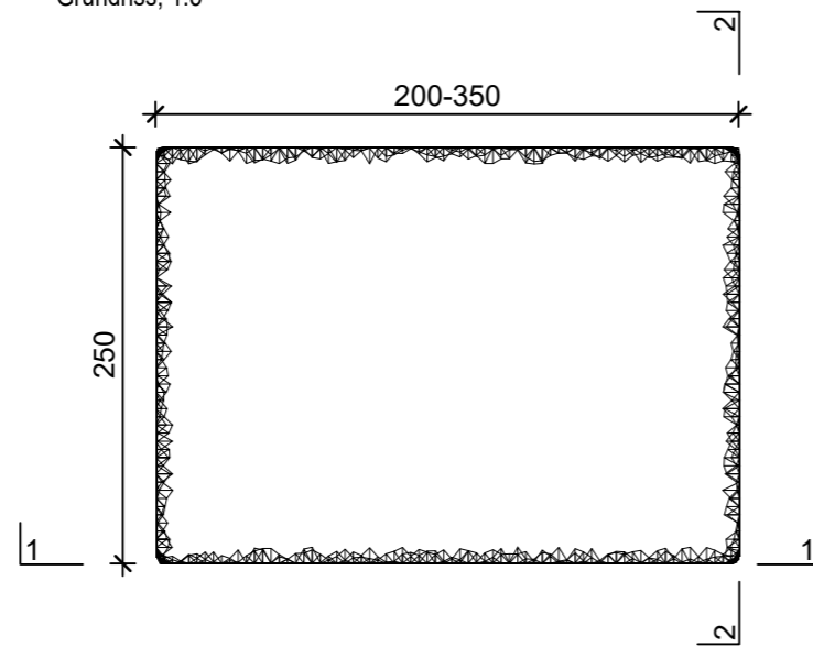
Grundriss, 1:5
