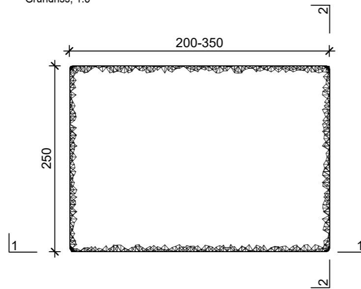
Grundriss, 1:5
