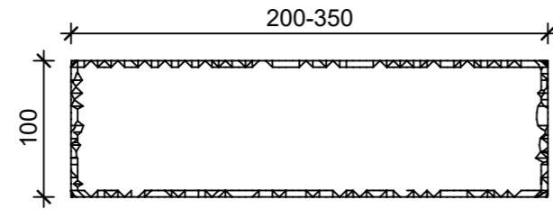
Schnitt 1-1, 1:5
