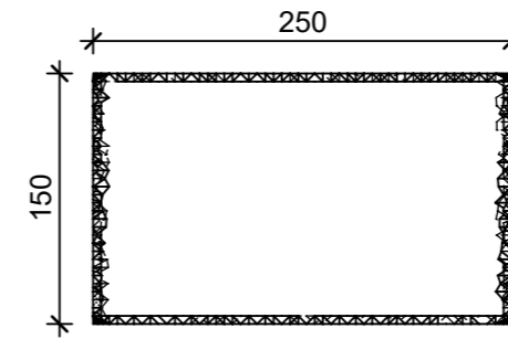
Schnitt 2-2, 1:5
