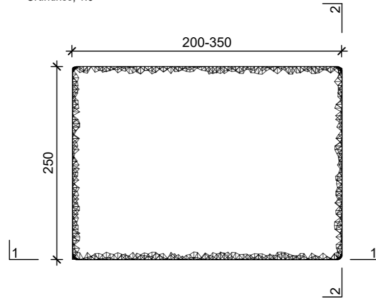
Grundriss, 1:5
