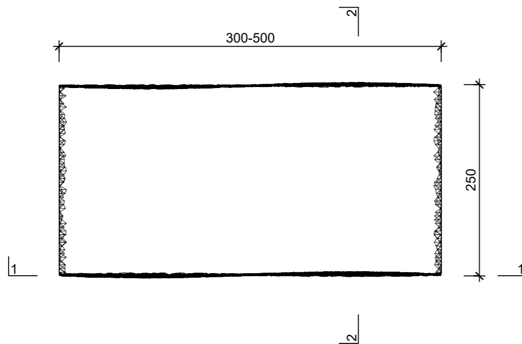
Grundriss, 1:5
