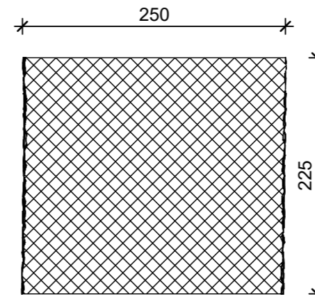
Schnitt 2-2, 1:5
