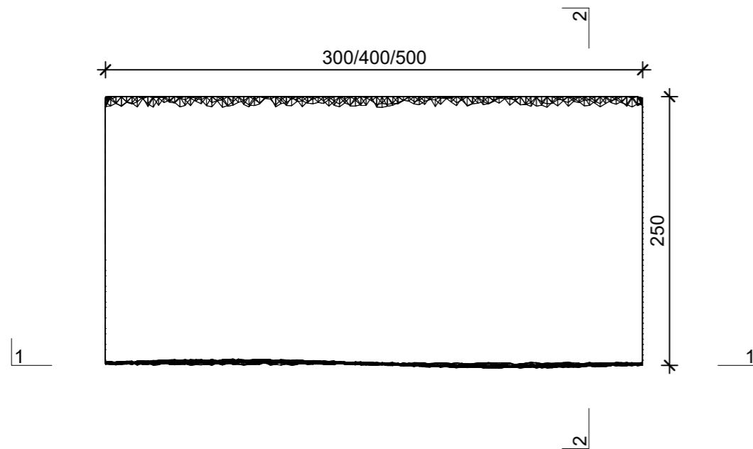
Grundriss, 1:5
