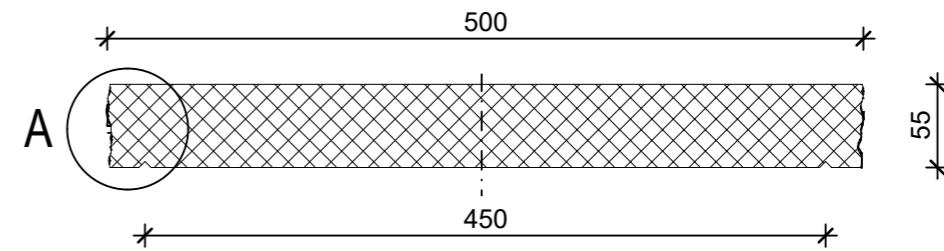
Schnitt 2-2, 1:5
