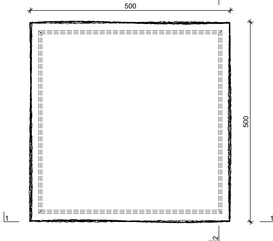
Grundriss, 1:5
