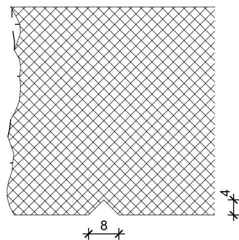
Detail A, 1:2
