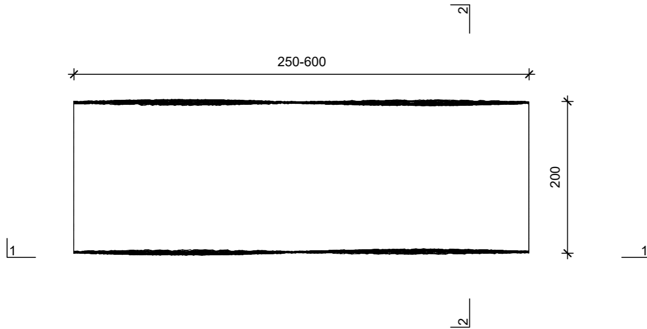
Grundriss, 1:5
