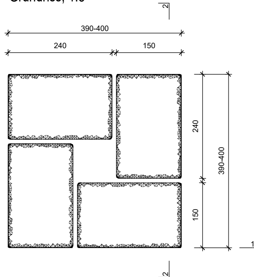
Grundriss, 1:5
