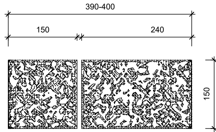
Schnitt 1-1, 1:5
