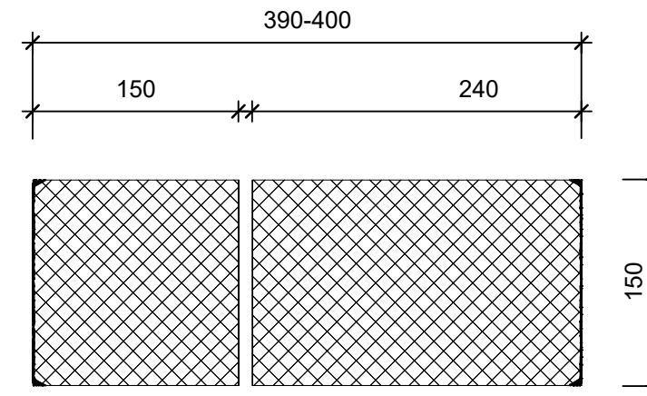
Schnitt 2-2, 1:5
