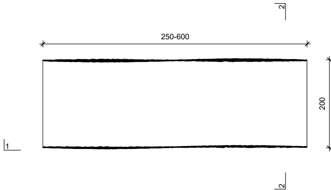
Grundriss, 1:5
