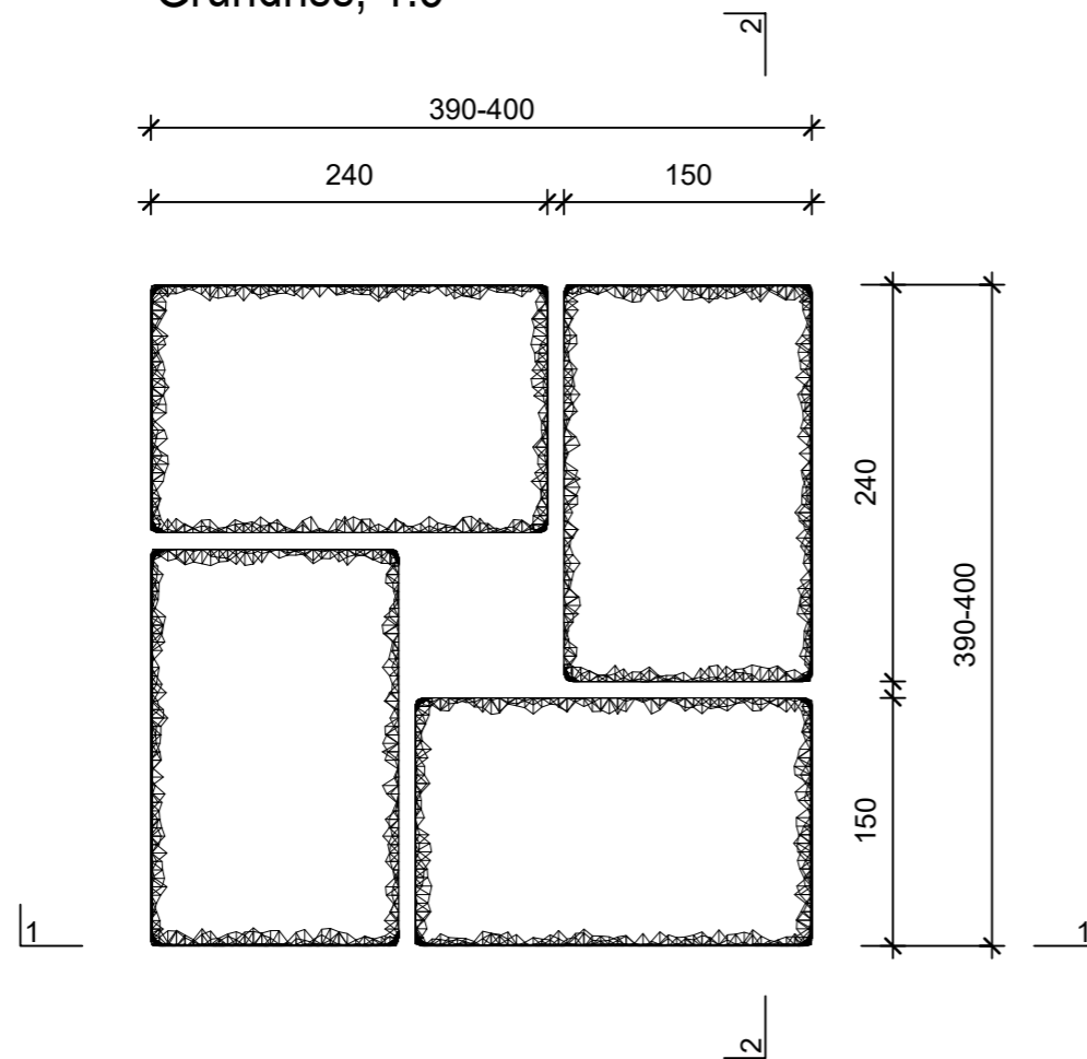
Grundriss, 1:5
