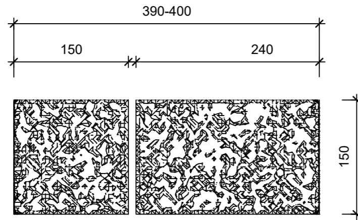
Schnitt 1-1, 1:5
