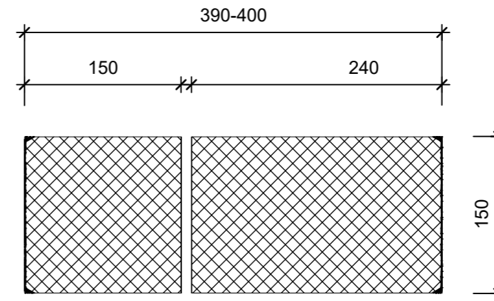
Schnitt 2-2, 1:5
