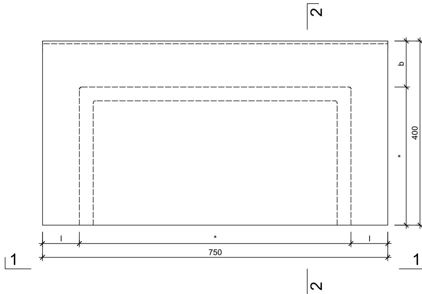
Grundriss, 1:5
