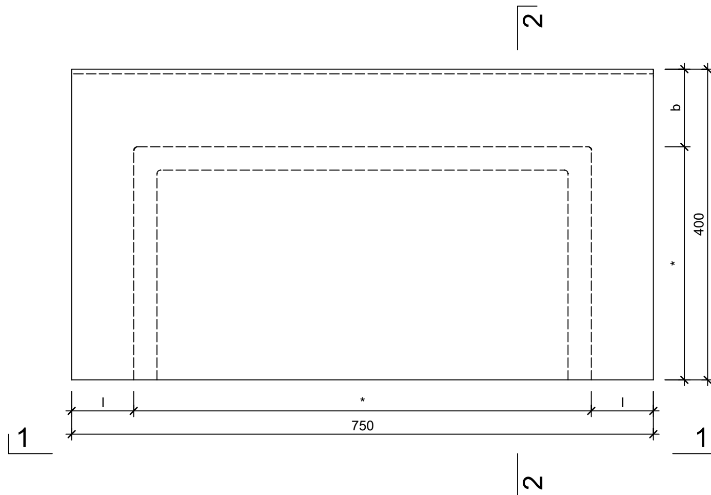
Grundriss, 1:5
