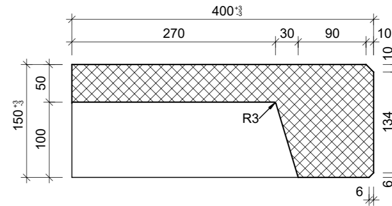
Schnitt 2-2, 1:5
