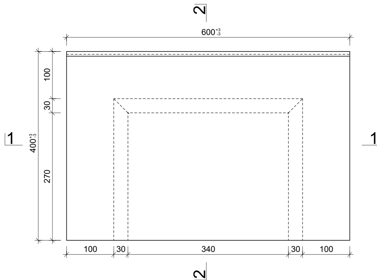
Grundriss, 1:5
