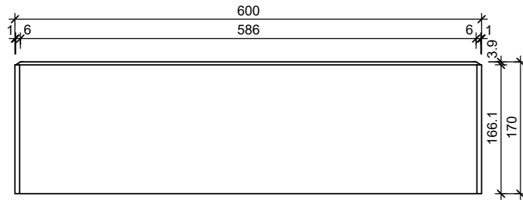
Grundriss, 1:5
