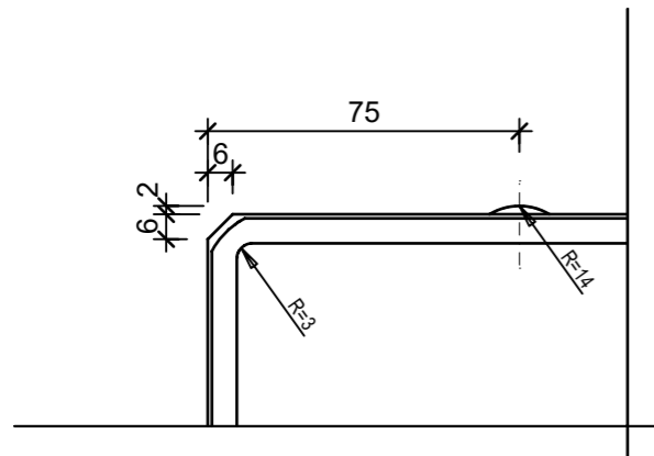
Detail A, 1:2
