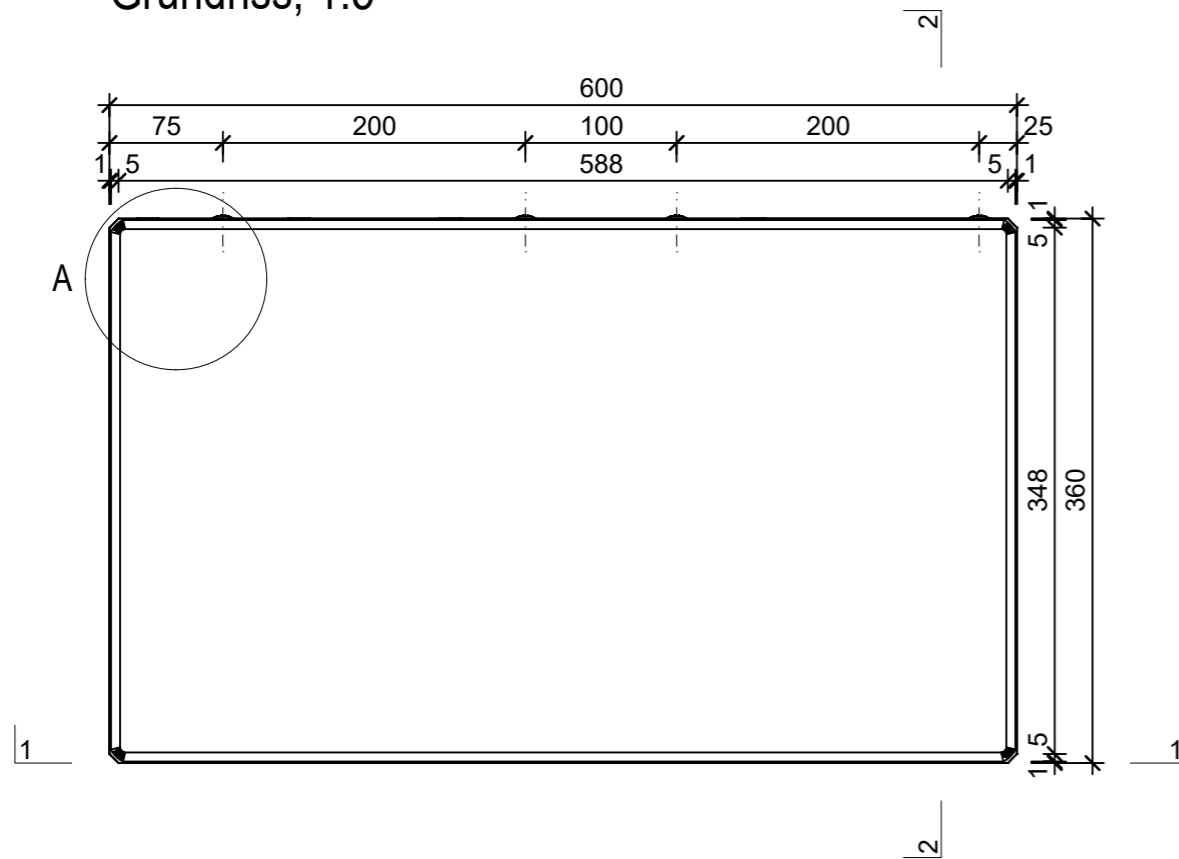
Grundriss, 1:5
