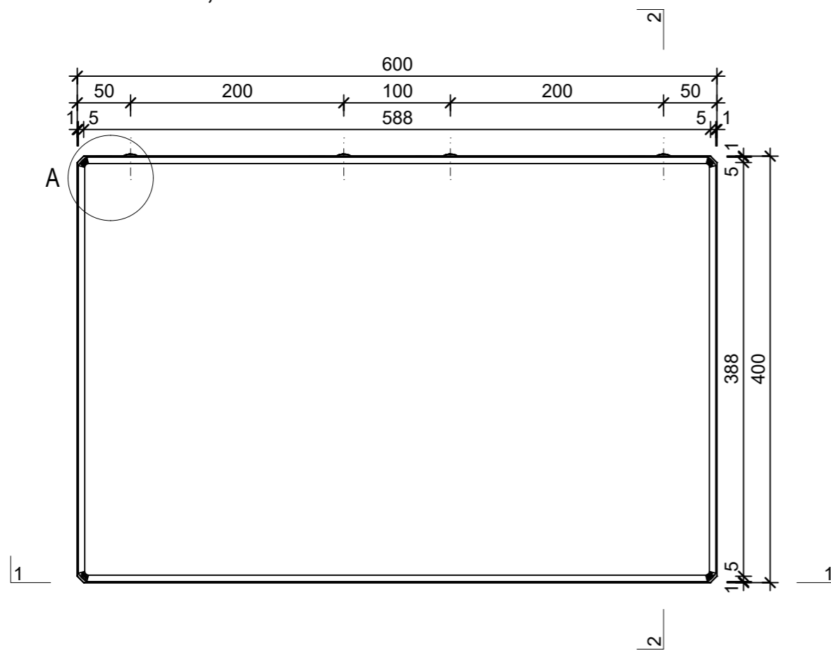
Grundriss, 1:5
