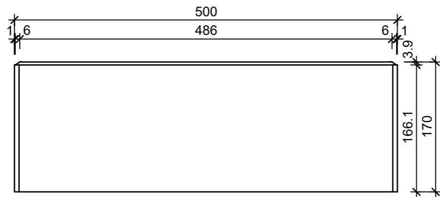
Grundriss, 1:5
