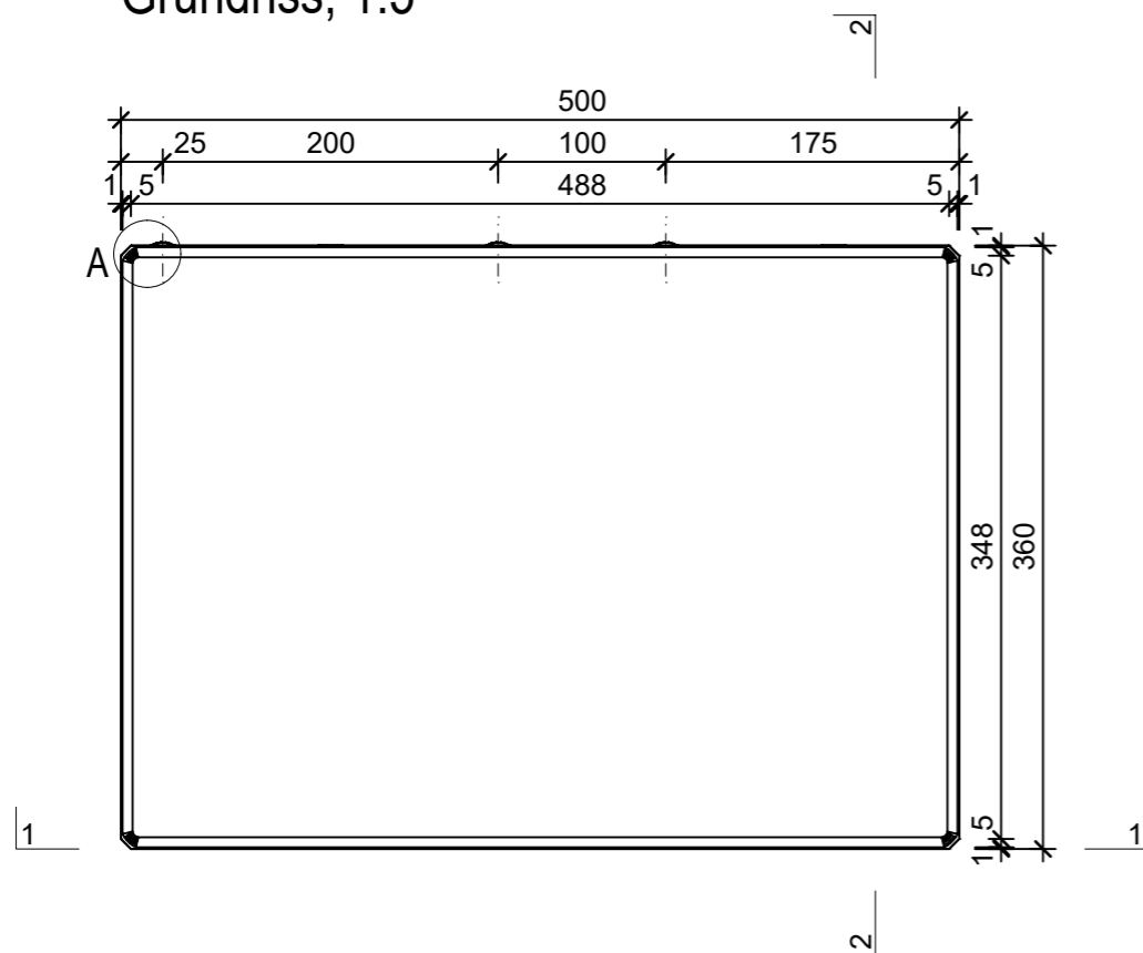
Grundriss, 1:5
