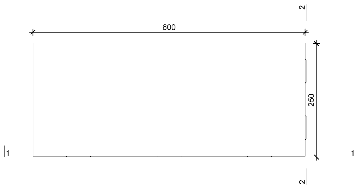
Grundriss, 1:5
