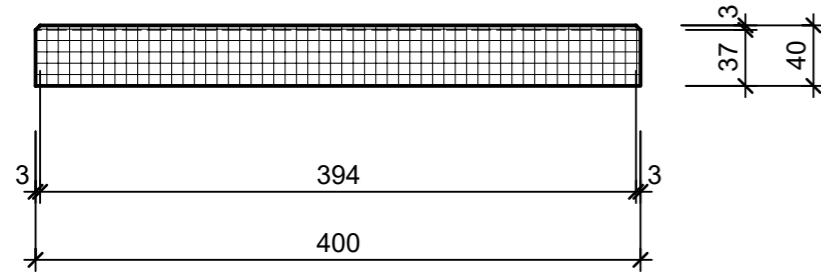
Schnitt 1-1 1:5
