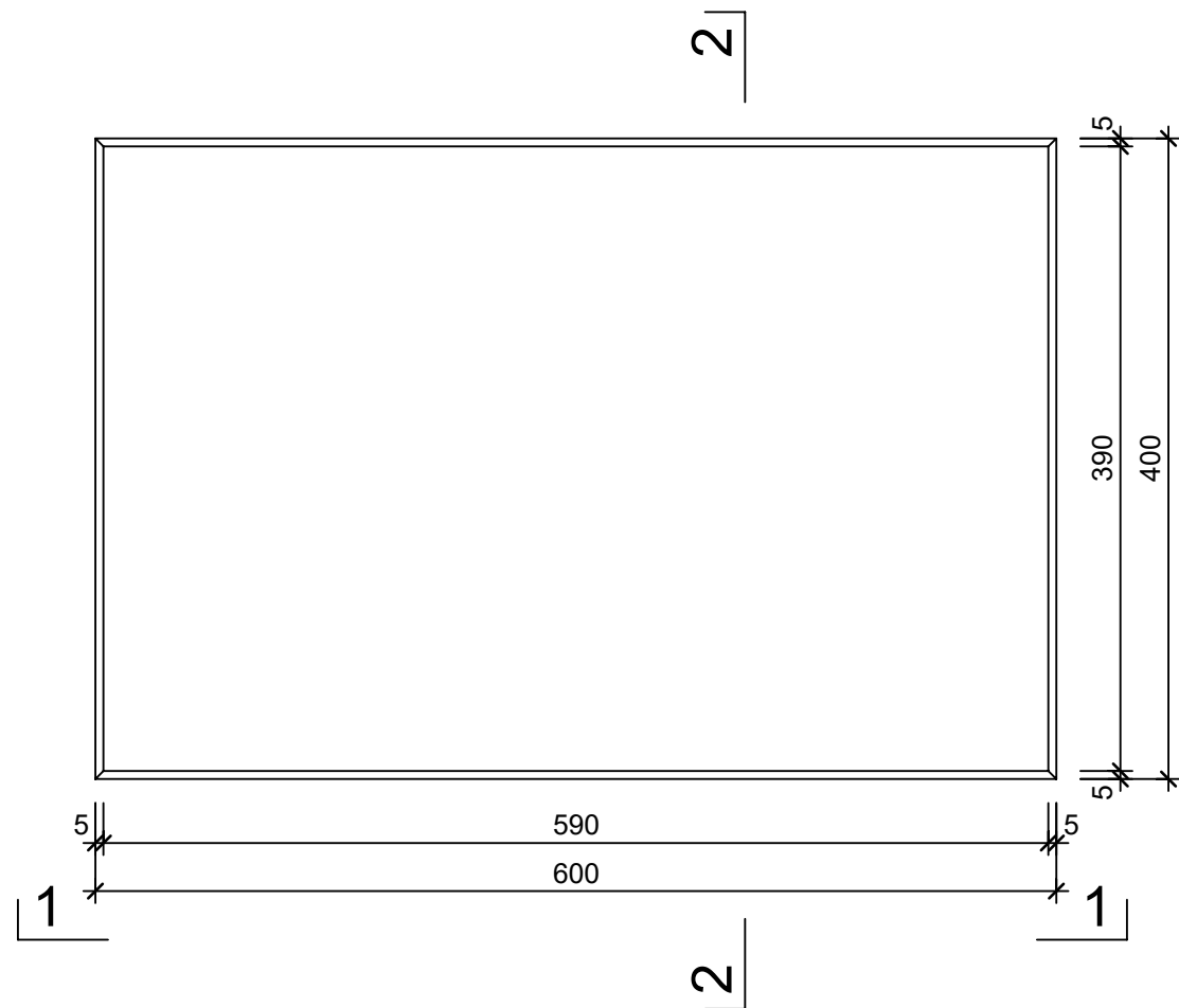
Grundriss, 1:5
