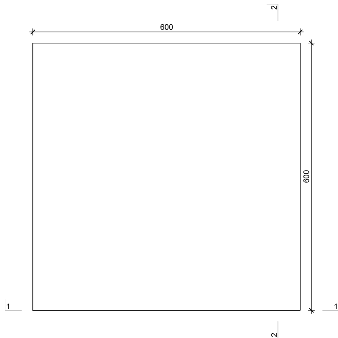
Grundriss, 1:5
