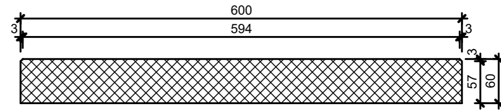
Schnitt 2-2, 1:5
