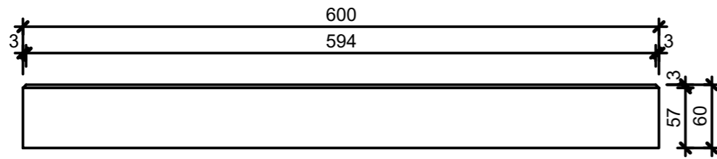
Schnitt 1-1, 1:5
