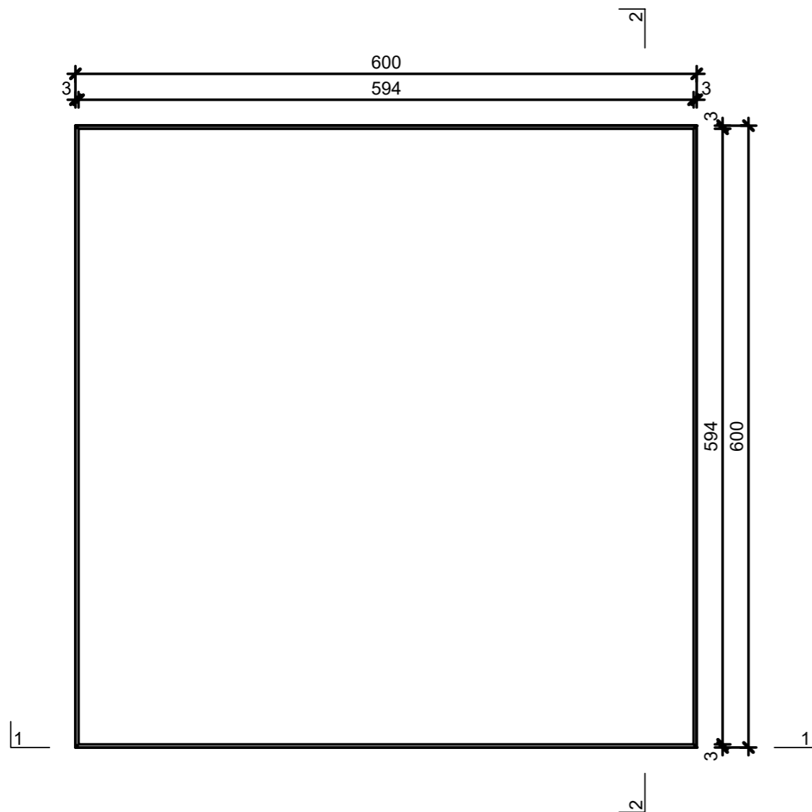
Grundriss, 1:5
