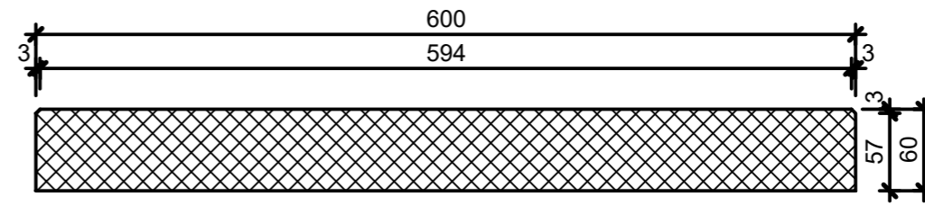
Schnitt 2-2, 1:5
