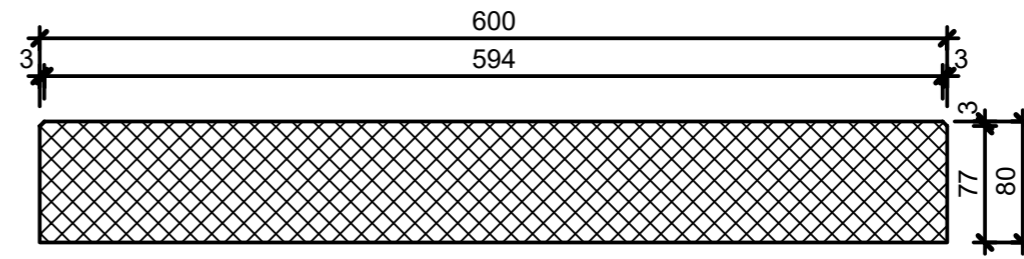
Schnitt 2-2, 1:5
