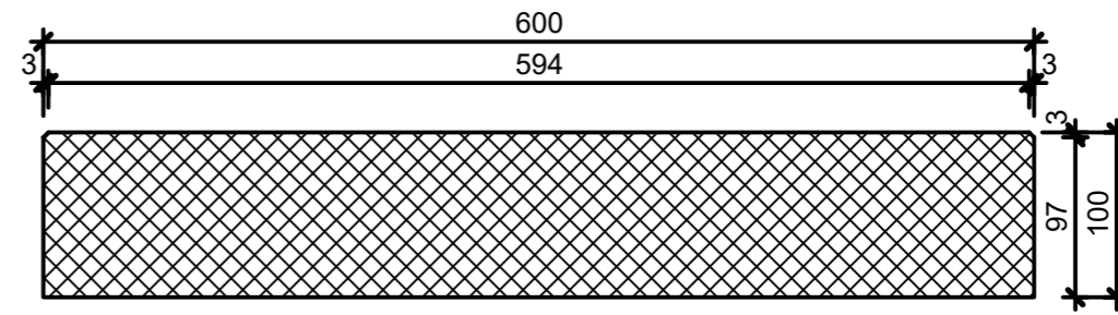
Schnitt 2-2, 1:5
