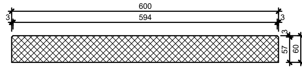
Schnitt 2-2, 1:5
