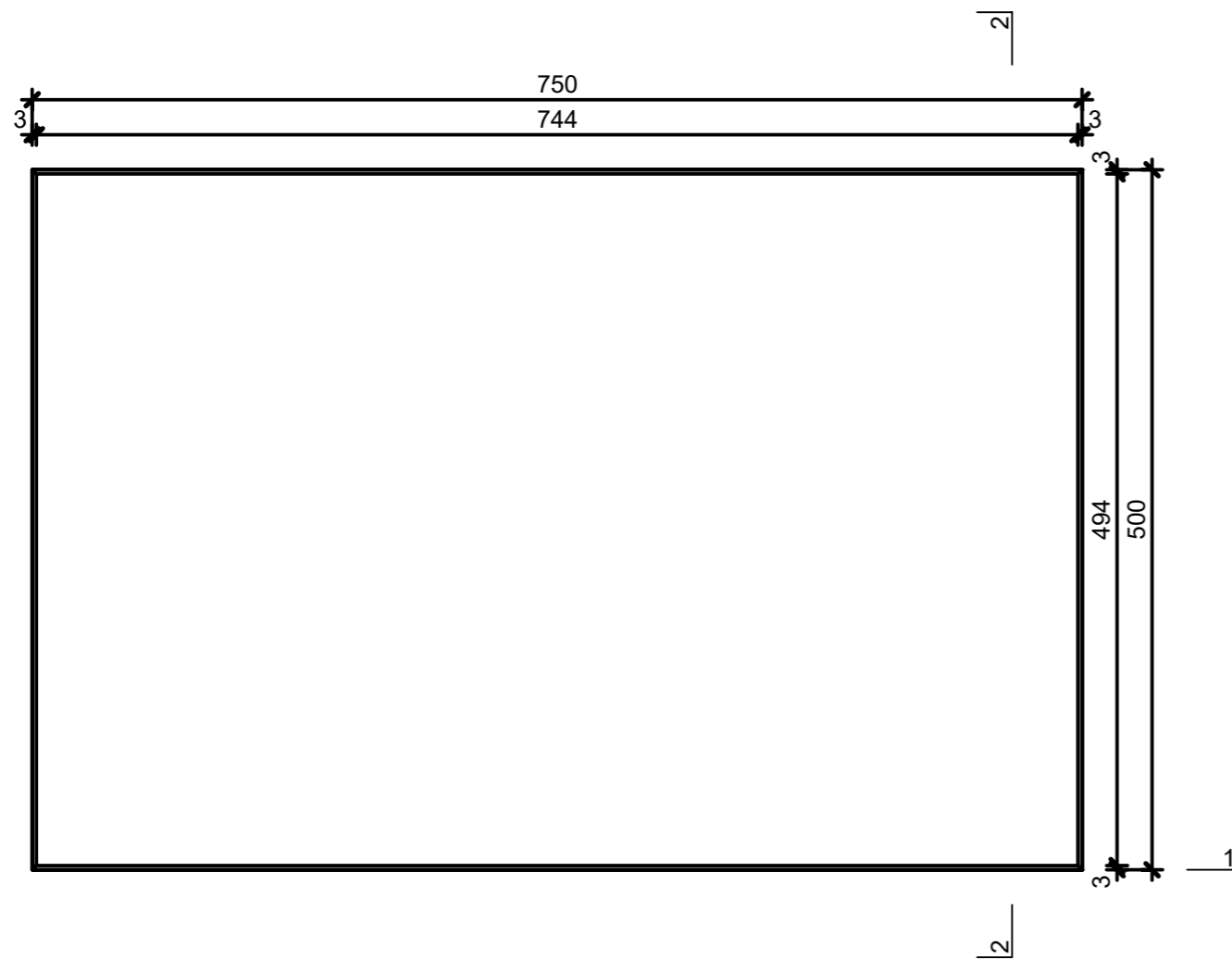
Grundriss, 1:5
