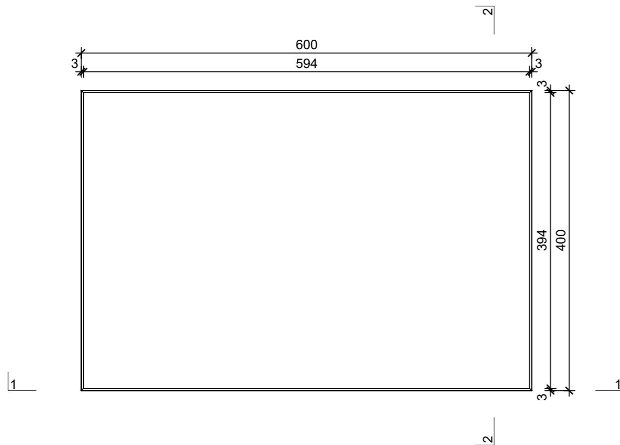
Grundriss, 1:5
