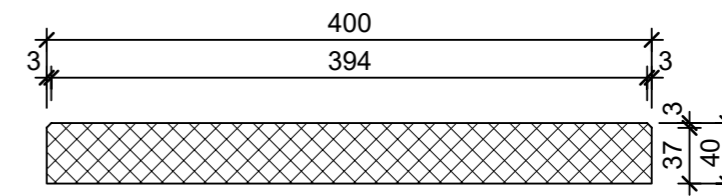
Schnitt 2-2, 1:5
