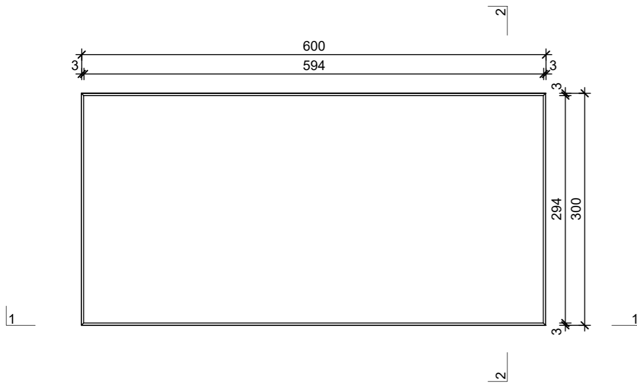
Grundriss, 1:5
