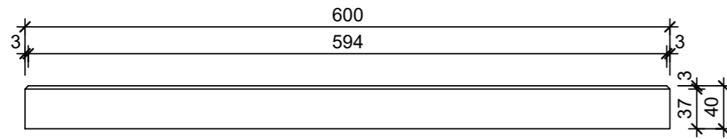
Schnitt 1-1, 1:5
