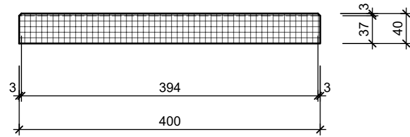
Schnitt 1-1 1:5
