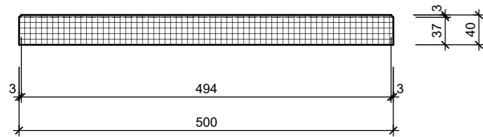
Schnitt 1-1 1:5
