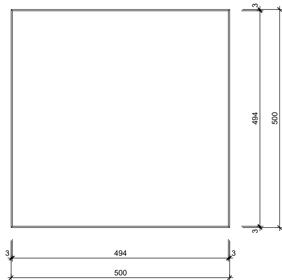
Grundriss 1:5
