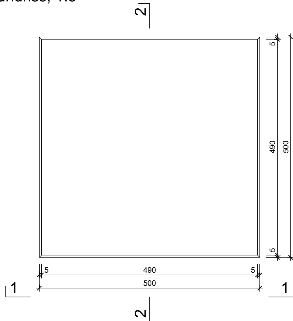
Grundriss, 1:5
