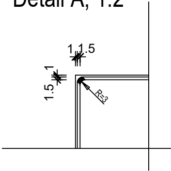
Detail A, 1:2
