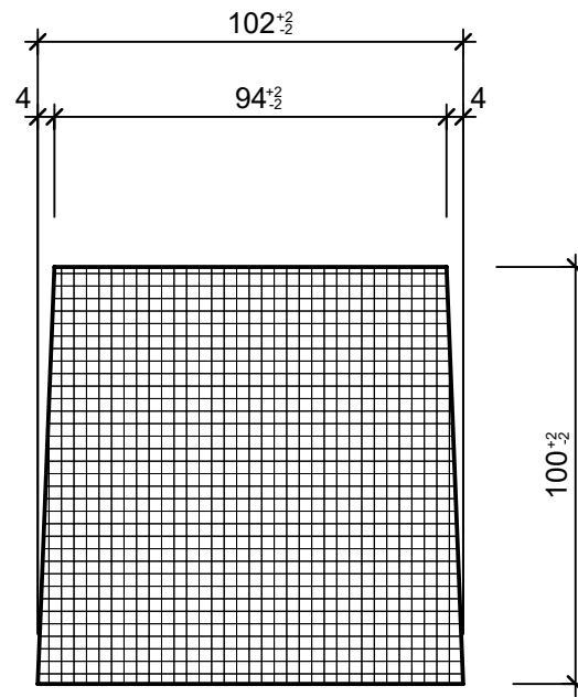
Schnitt A-A, 1:2
