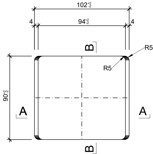
Grundriss, 1:2
