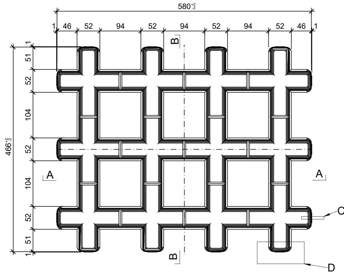
Grundriss, 1:5
