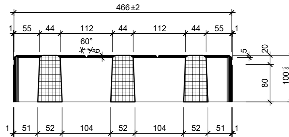
Detail D, 1:2
