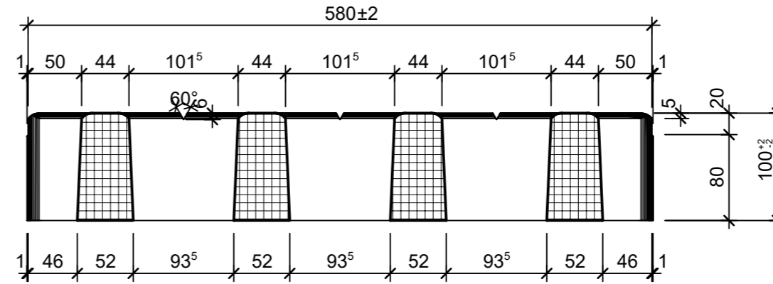
Schnitt B-B, 1:5
