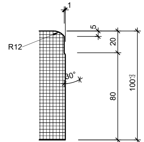
Detail C, 1:2
