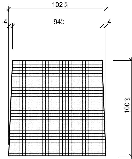
Schnitt A-A, 1:2
