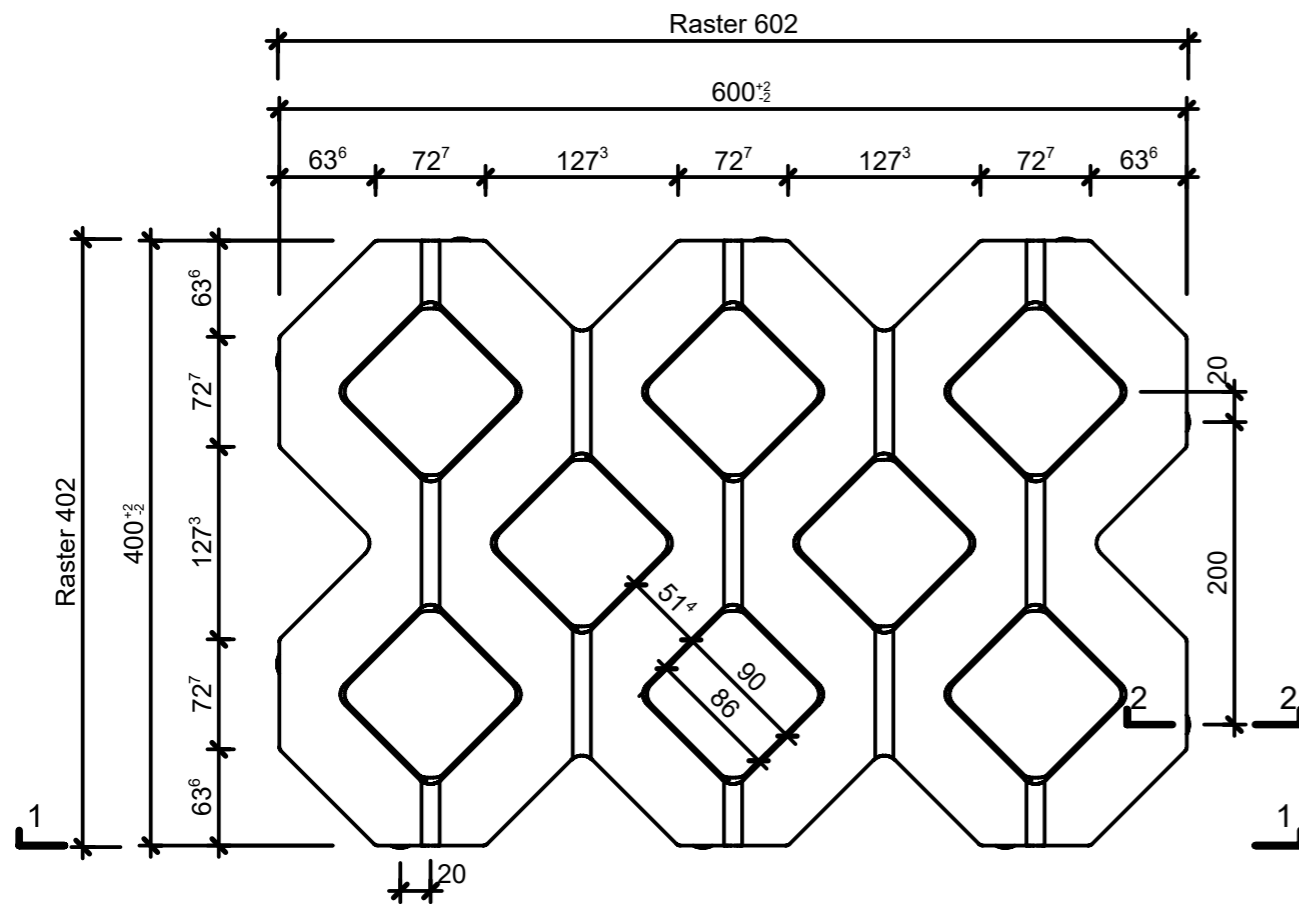
Grundriss 1:5
