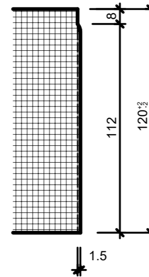
Schnitt 2-2, 1:2
