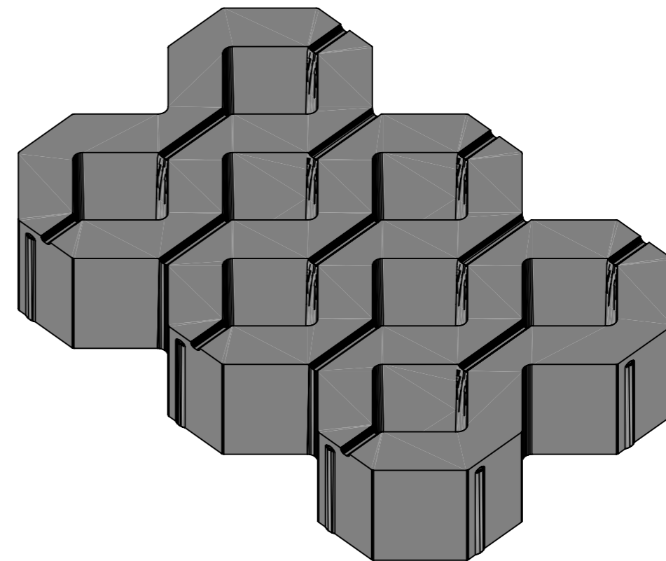
Isometrie 1:5
