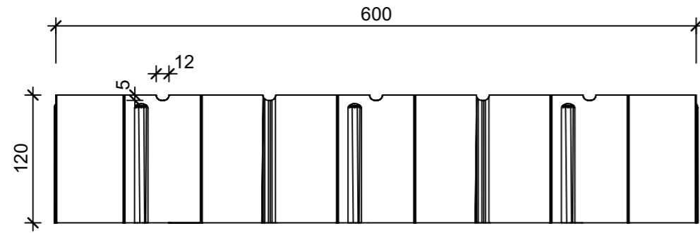
Schnitt 1-1, 1:5
