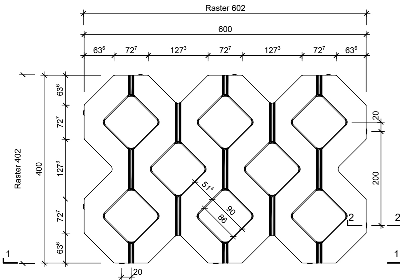
Grundriss 1:5
