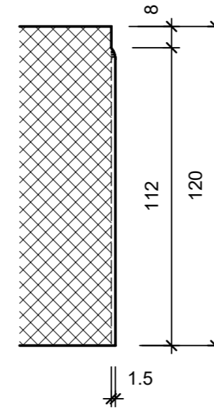
Schnitt 2-2, 1:2
