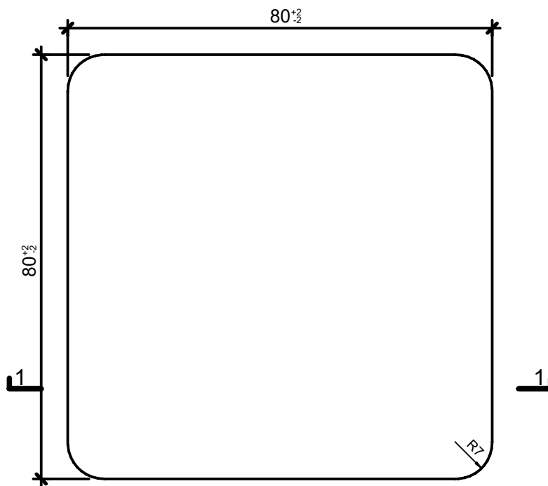
Grundriss 1:1
