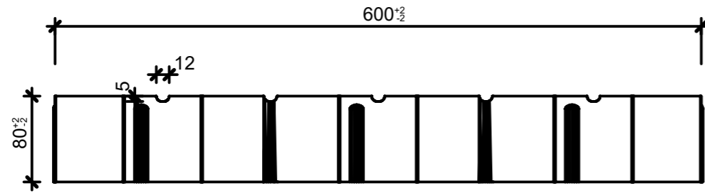
Schnitt 1-1, 1:5
