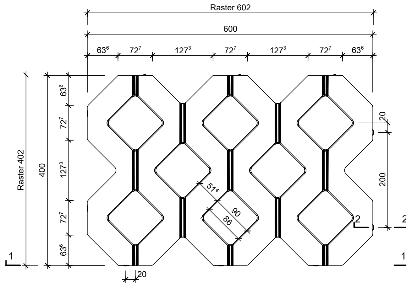
Grundriss 1:5
