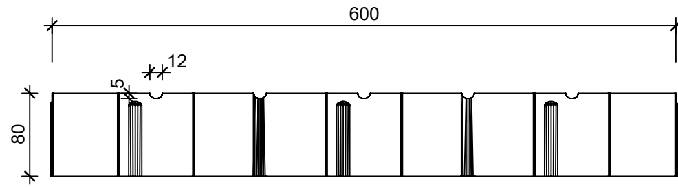
Schnitt 1-1, 1:5
