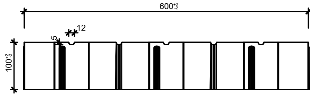
Schnitt 1-1, 1:5
