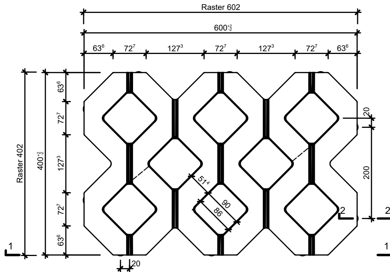
Grundriss 1:5
