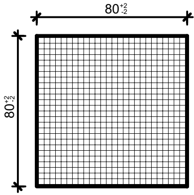
Schnitt 1-1, 1:2
