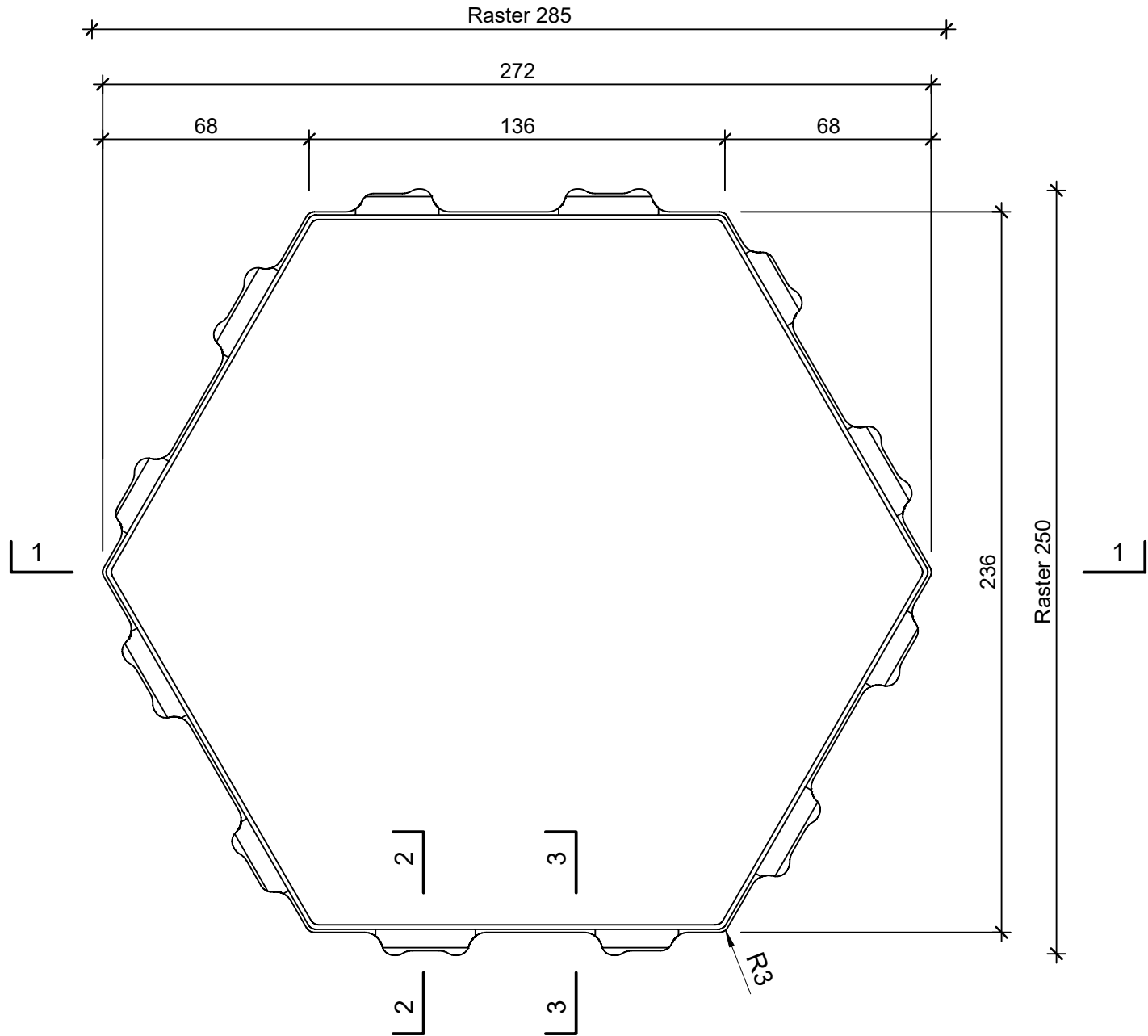
Grundriss 1:2
