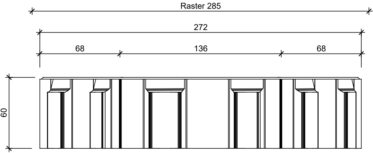
Schnitt 1-1, 1:2
