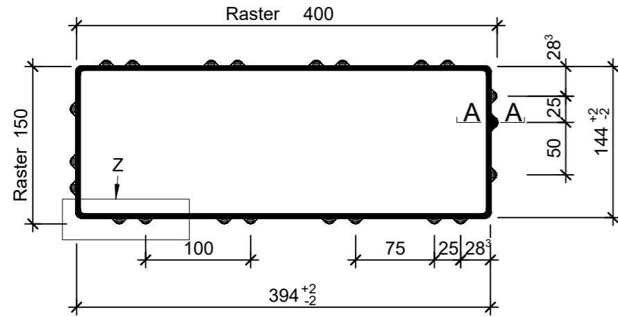
Grundrisse, 1:5
