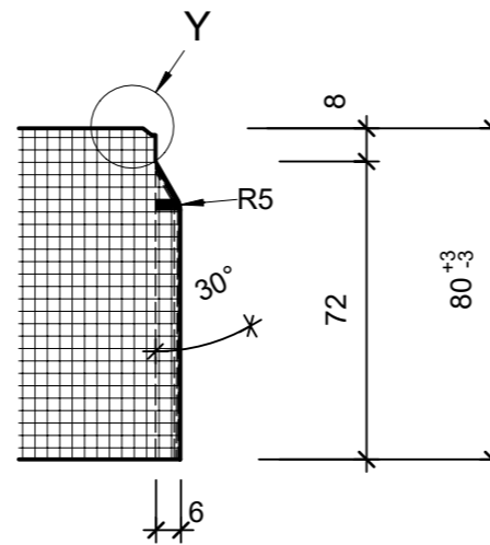
Schnitt A-A, 1:2
