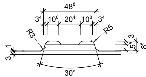
Detail C, 1:2
