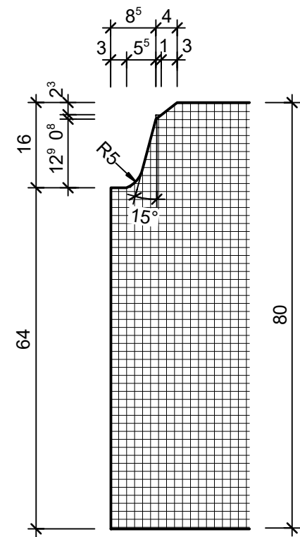
Detail A, 1:1
