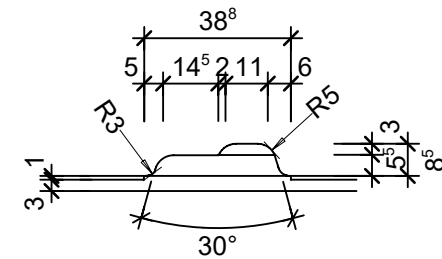
Detail C, 1:2
